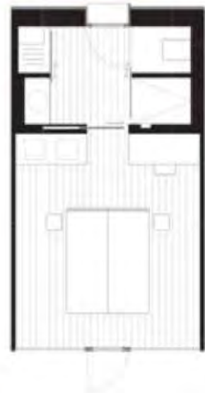
Grundriss eines Hotelzimmers
